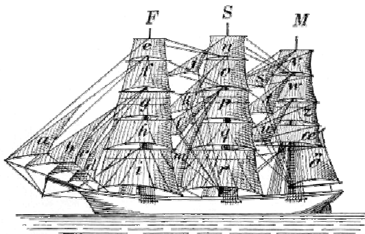
Fig. 247. Benævnelse paa Master og Sejl.
